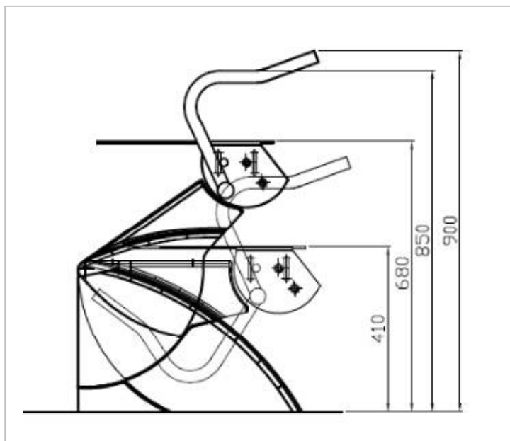
Option – rabatable Griffe Artikel Nr. 8141400
