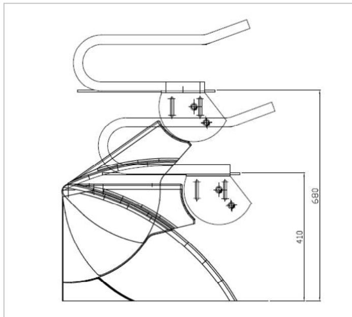
Option – fixe Griffe Artikel Nr. 8141300
